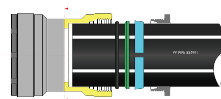
การจัดเรียงชิ้นส่วน ติดตั้งท่อพีซี 150 - 250 มม.
