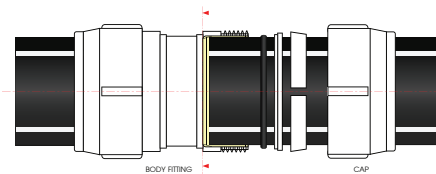
การจัดเรียงชิ้นส่วน ติดตั้งท่อพีซี 40 - 100 มม.
