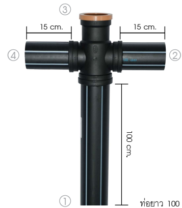
ท่อยาว 100 ซม.
