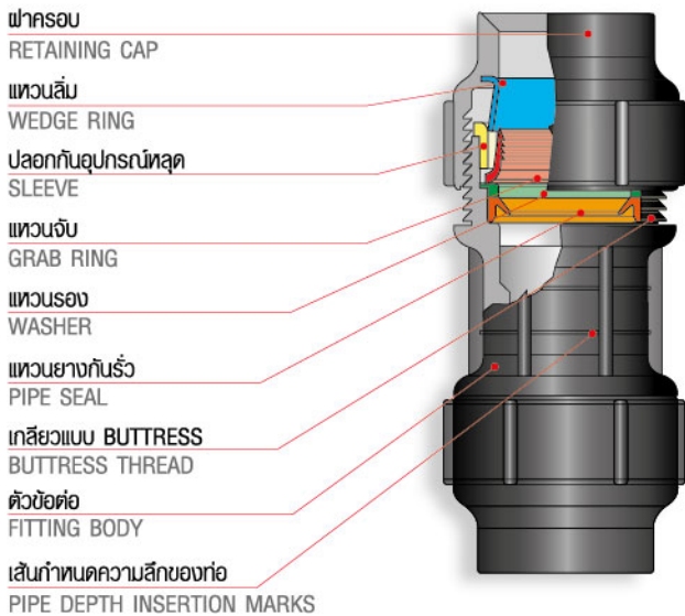
ส่วนประกอบข้อต่อระบบสวมล๊อค FEATURES OF GRAB LOCK FITTING SYSTEM
